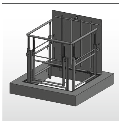
Integriertes, klappbares und ausziehbares Geländer in HS12 Built-in, fold-out and extendable guard rail in an HS12
